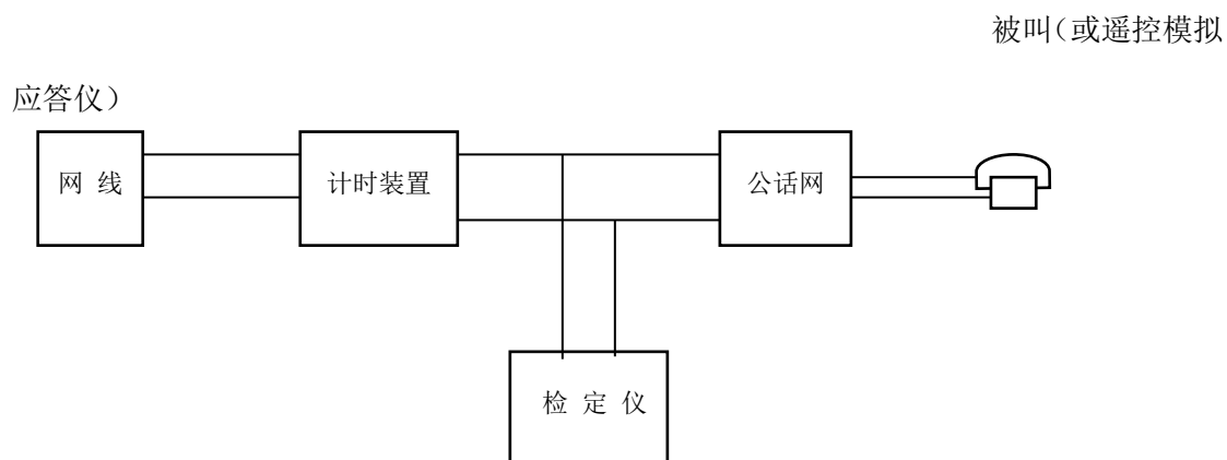
图 1 并联接入法连接示意图
