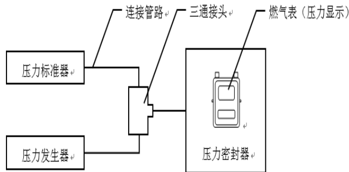
图3 压力传感器检定示意图
