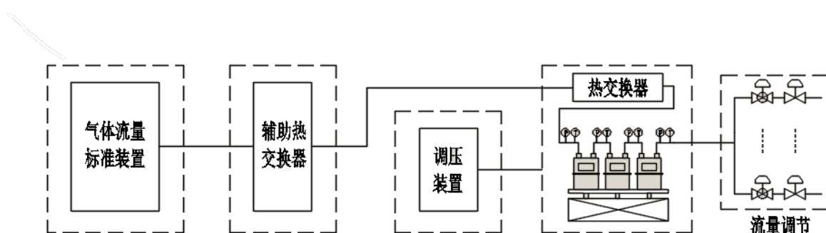
图 4 总量法检定试验设备示意图
