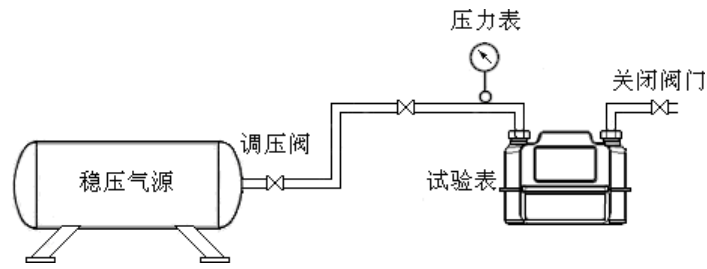
图1 密封性试验示意图
